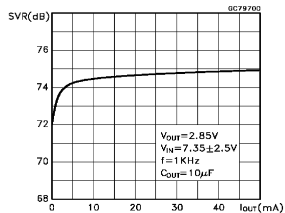
S.V.R. vs Output Current
