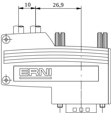
Kabelanschluss vertikal cable entry vertical
