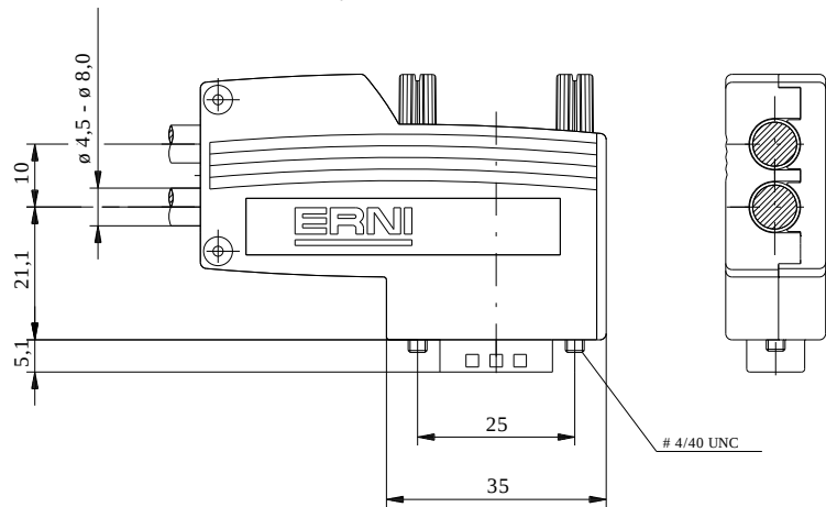
Kabelanschluss horizontal cable entry horizontal
