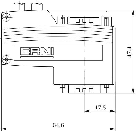
Kabelanschluss vertikal mit Serviceanschluss und Schalter cable entry vertical with PU connection and switch
