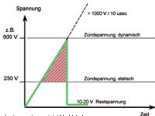
Verhalten eines 230V-Ableiters
