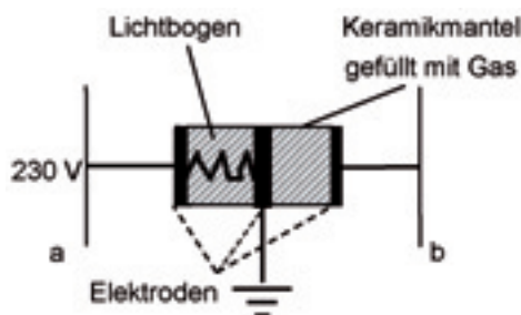
Dreipol-Ableiter
