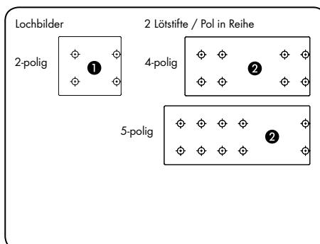
① Blindstück entsprechend 1 x Rastermaß ② Blindstück entsprechend 2 x Rastermaß
