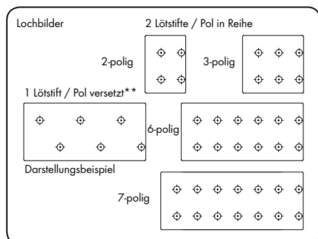
** Ausführungen mit versetzten Lötstiften zur Erhöhung der Luft- und Kriechstrecken auf Anfrage
