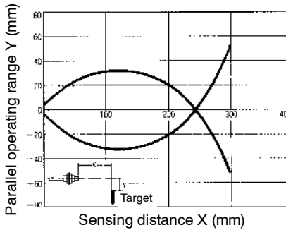
E32-D51 with E3X-NH amplifier
