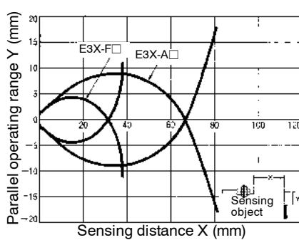
E32-D61 with E3X-A and E3X-F amplifiers
