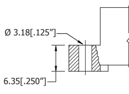
FLUSH MOUNTING (D)
