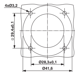
Einbaumaße
