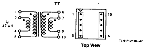
FIGURE 27. Schott 26606
