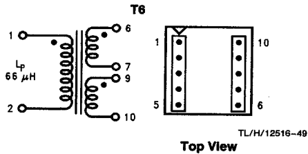
FIGURE 28. Schott 67140900
