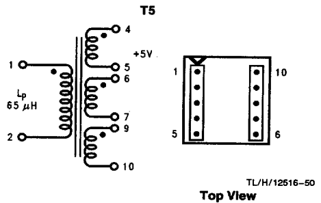
FIGURE 29. Schott 67140890
