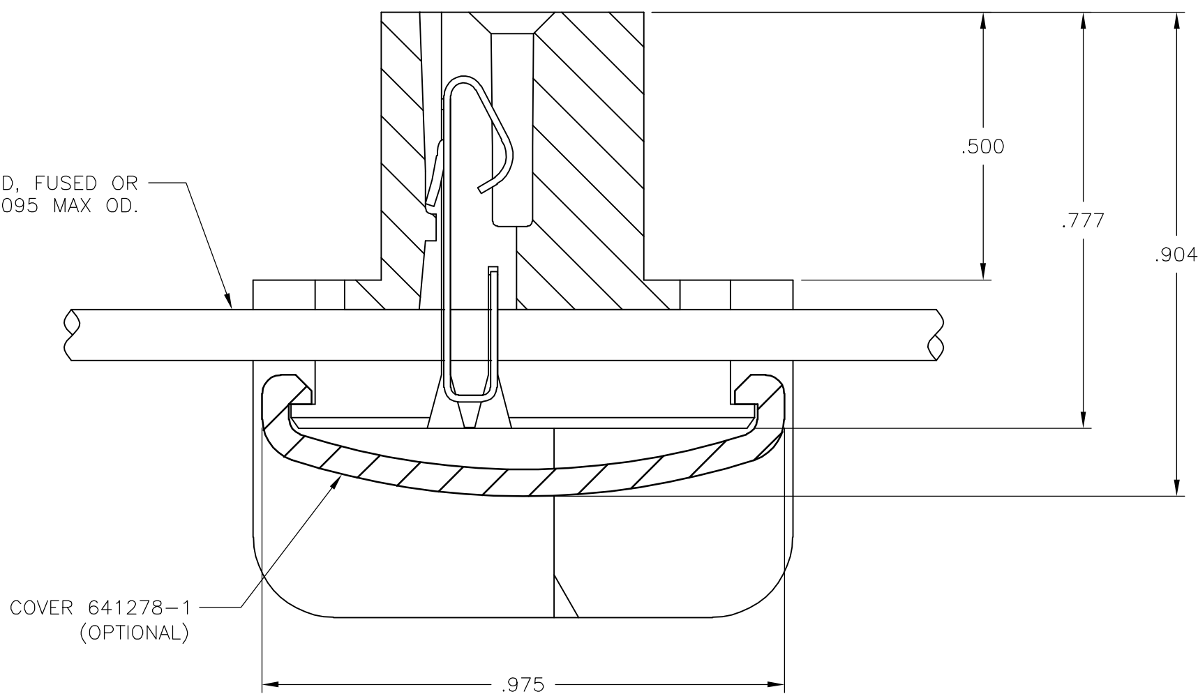
MTA SECTION
