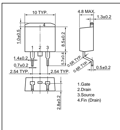
3) TO-263 (MP-25ZJ)
