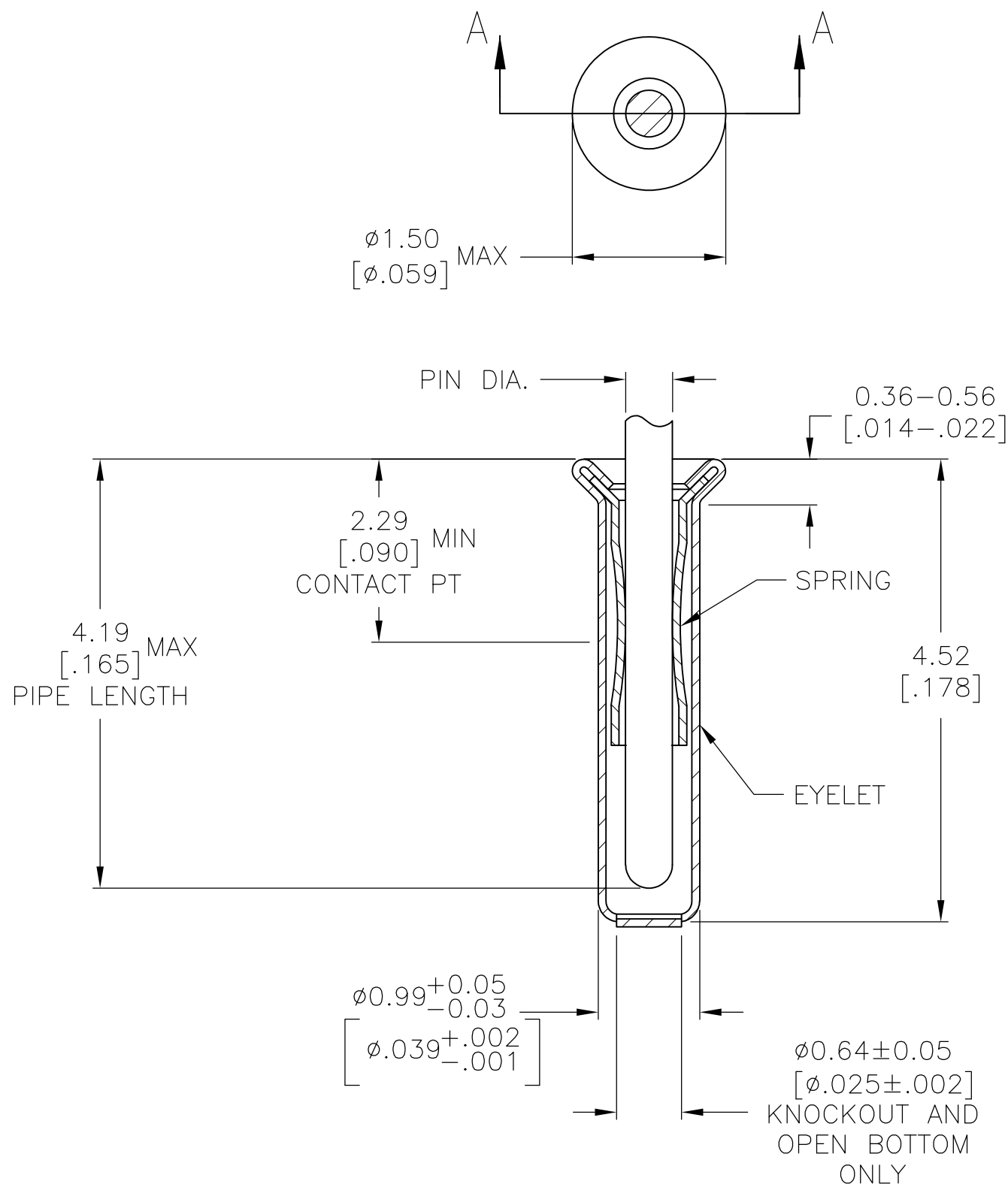
SECTION A-A
