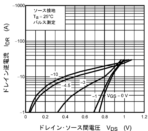
図 8.7 I_D - V_{DS}
