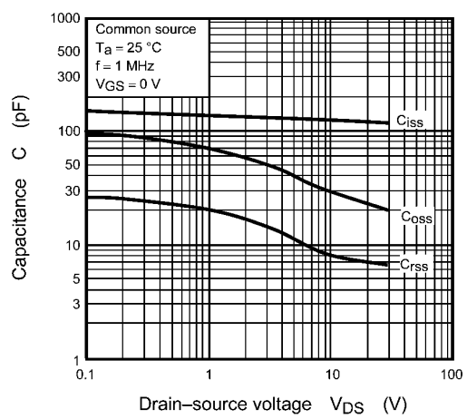
Fig. 7.10 C - V_{DS}
