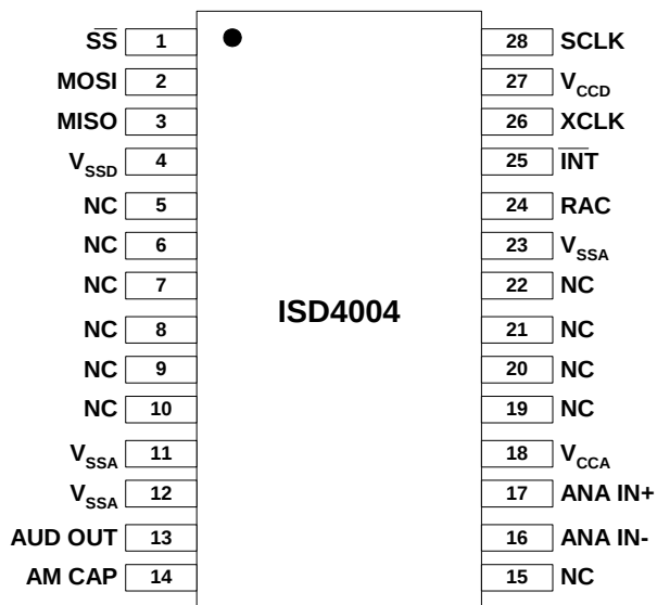
SOIC / PDIP
