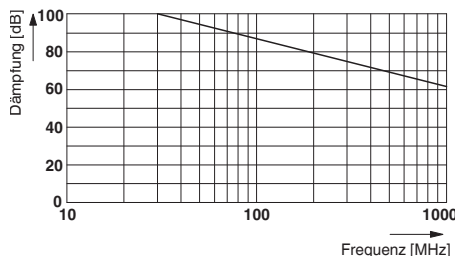
Schirmdämpfungskurve Serie RC in Anlehnung an DIN EN 50289-1-6
