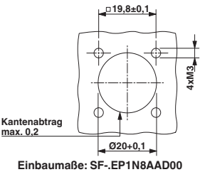
Einbaumaße: SF-EP1N8AAD00
