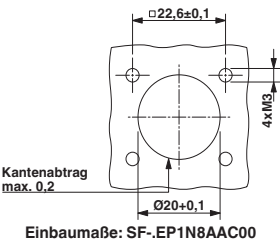
Einbaumaße: SF-EP1N8AAC00
