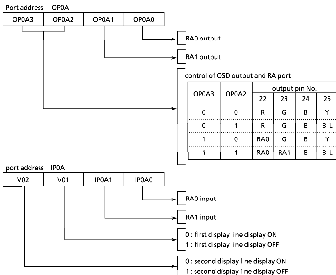
Figure 3-8. Port RA
