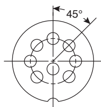
8 Pin 270 Arc 171-1080-E 171-1081-E
