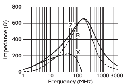
BLA31AG601SN4
