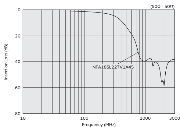
NFA18SL227V1A45
