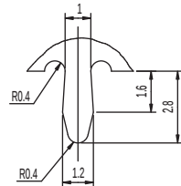
K DETAIL 2:1
