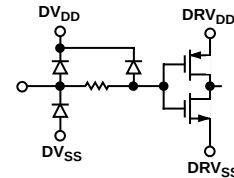
c) CLK
