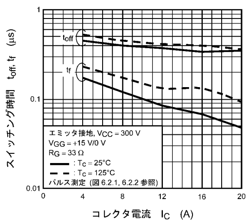
図 8.10 t_{off} , t_f - I_C
