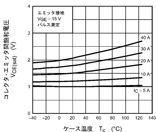
図 8.6 V_{CE(sat)} - T_C
