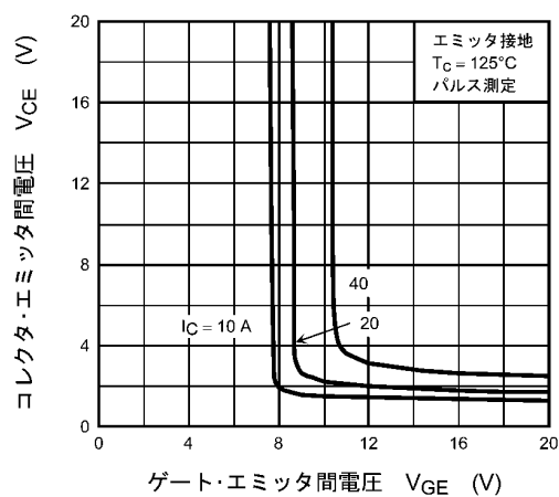
図 8.4 V_{CE} - V_{GE}
