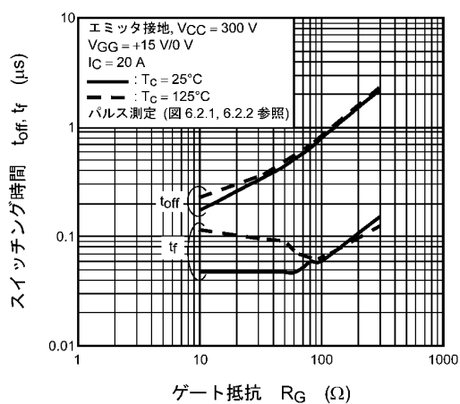
図 8.9 t_{off} , t_f - R_G
