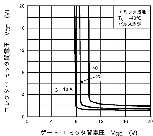
図 8.2 V_{CE} - V_{GE}
