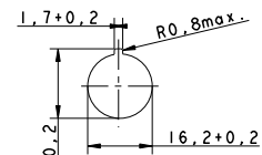
Einbauöffnung
