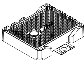
ACEPACK™ 2
