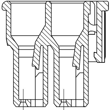
SECT A-A
