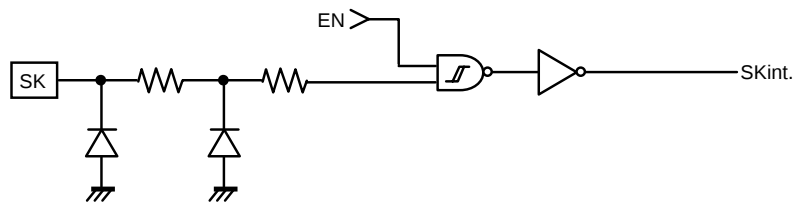
Figure 38. Input Circuit (SK)
