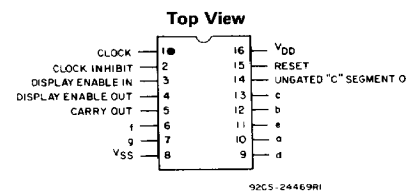
CD4026B
