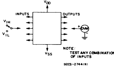
Fig. 16 – Input voltage.
