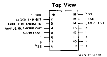
CD4033B
