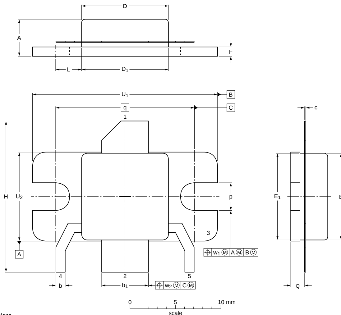
Dimensions
