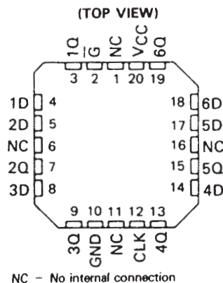
SN54LS378 . . . FK PACKAGE
