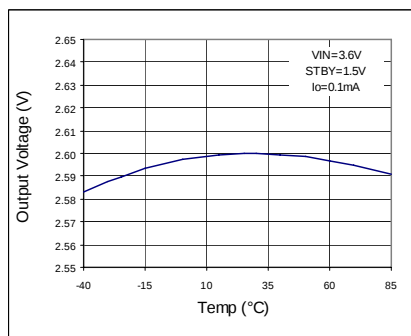
Fig 138. VOUT - Temp
