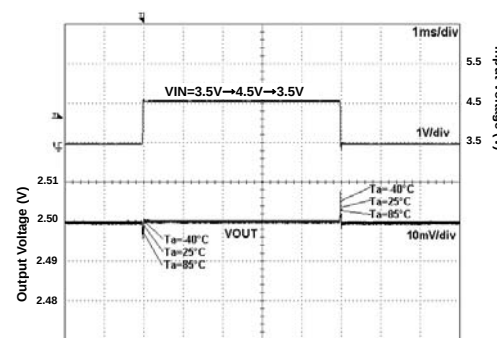
Fig 128. VIN Response
