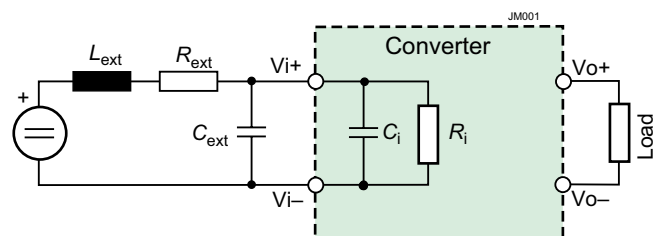
Fig. 8 Input configuration
