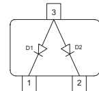
BAS40-06 BAS40-06W
