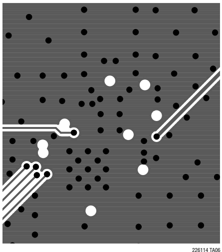
Inner Layer 3
