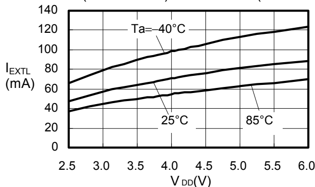
(6) I_{EXTL}-V_{DD}
