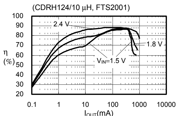
(16) S-8341C25AFT
