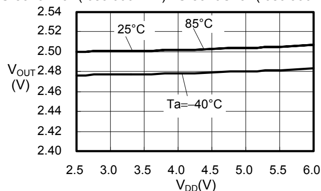
(10) V_{OUT}-V_{DD}
