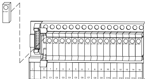
G7TC-OC16
