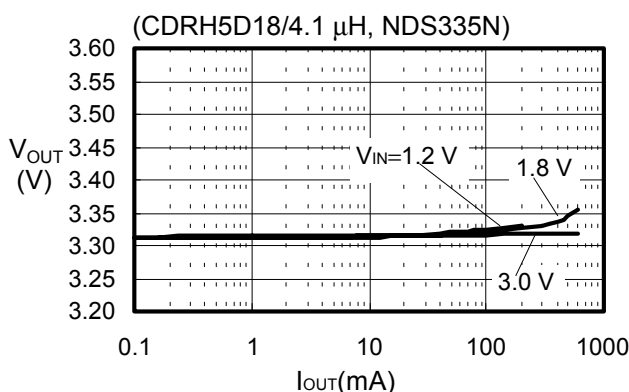
(7) S-8341A33AFT
