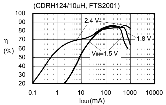
(4) S-8341A25AFT
