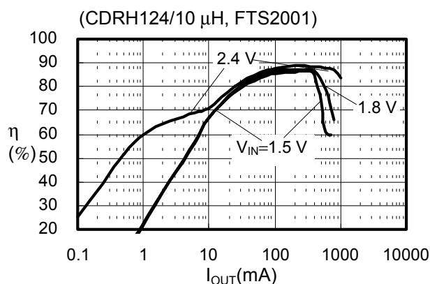
(16) S-8341C25AFT
