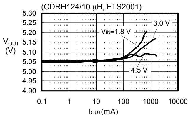
(12) S-8341A50AFT
