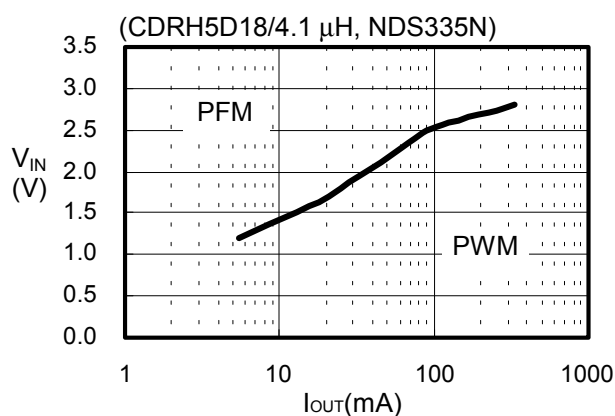
(29) S-8341A50AFT
