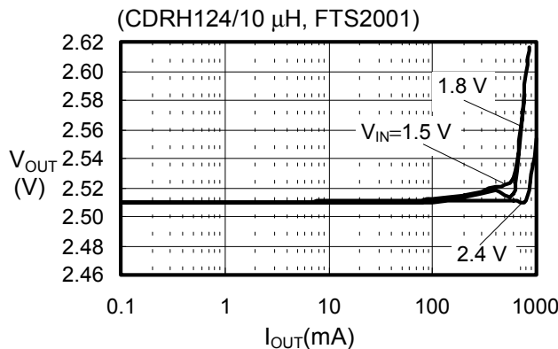
(16) S-8341C25AFT
