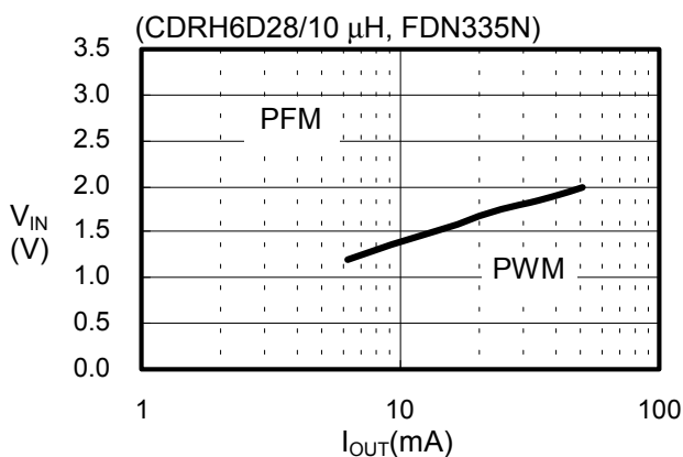
(31) S-8341C25AFT
