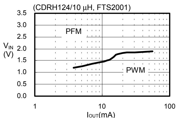
(28) S-8341A33AFT
