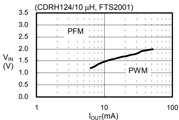
(32) S-8341C25AFT
