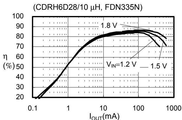
(15) S-8341C25AFT
