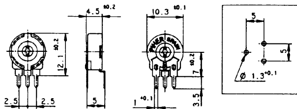
PT 10 Lh (5) PTC 10 Lh (5)
