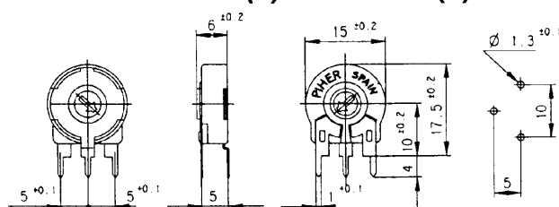
PT 15 Lh (5) PTC 15 Lh (5)
