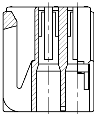
Seccion B-B SECTION
