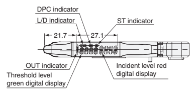
DIN track mounting
