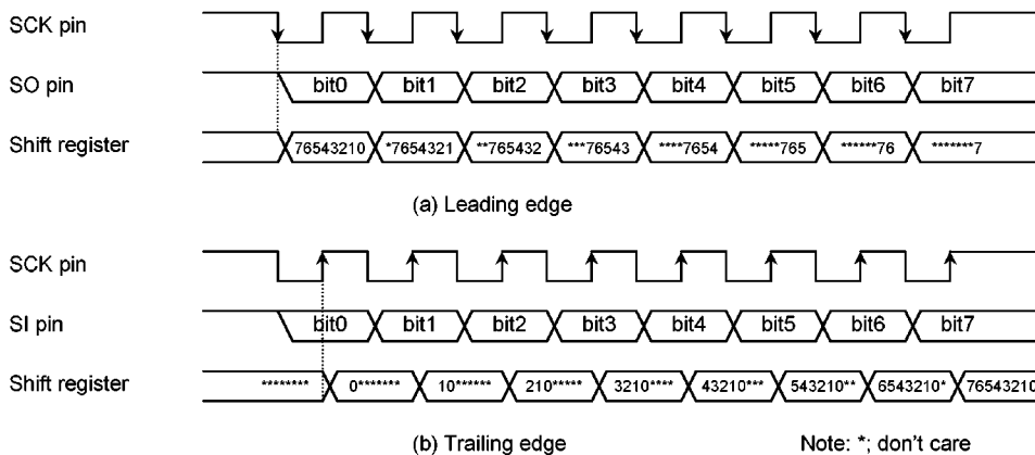
Figure 3.16.4 Shift Edge
