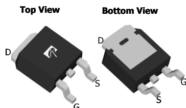
TO252 DPAK
