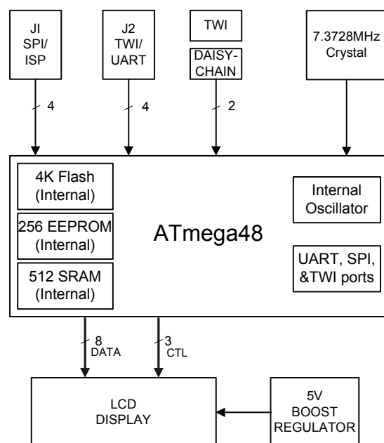
PmodCLS Block Diagram
