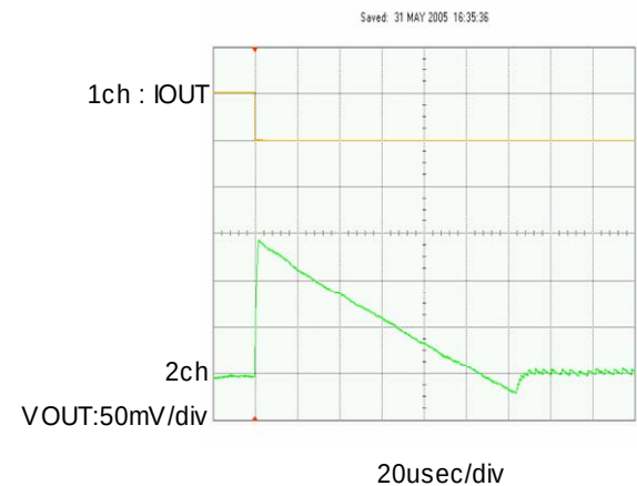
IOUT=300m A \rightarrow 1m A
