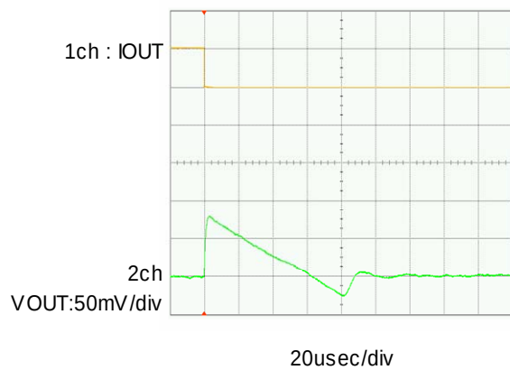
IO UT =100m A → 1m A
