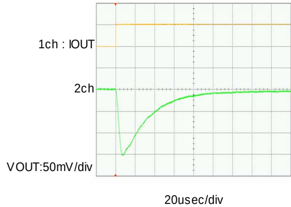
IO UT =1m A → 300m A
