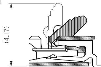
アクチュエータを開いた状態
