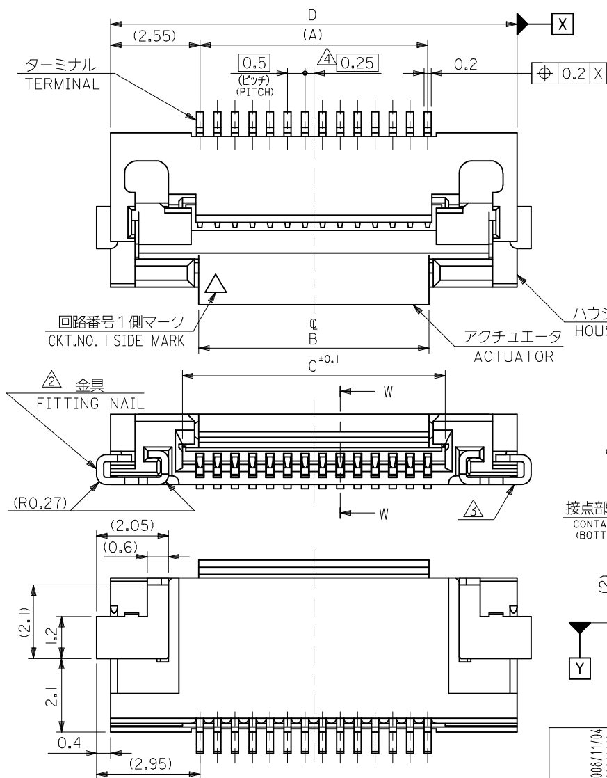
アクチュエータを開いた状態
