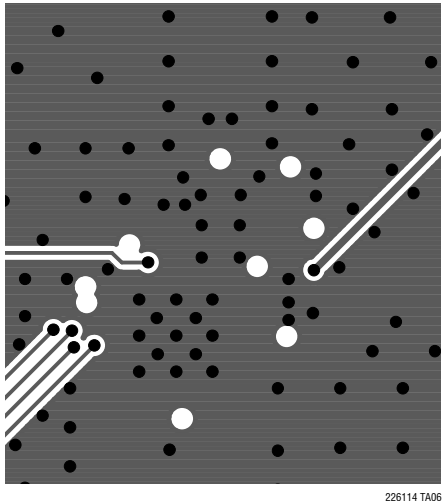
Inner Layer 3
