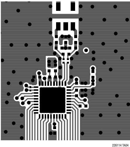
Top Side
