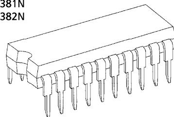
SDIP20-P-300-1.78
