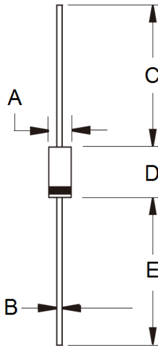
DO-204AL (DO-41)
