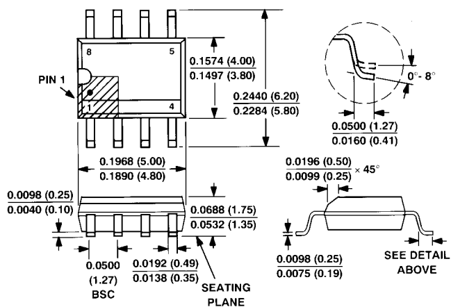
SOIC-8
