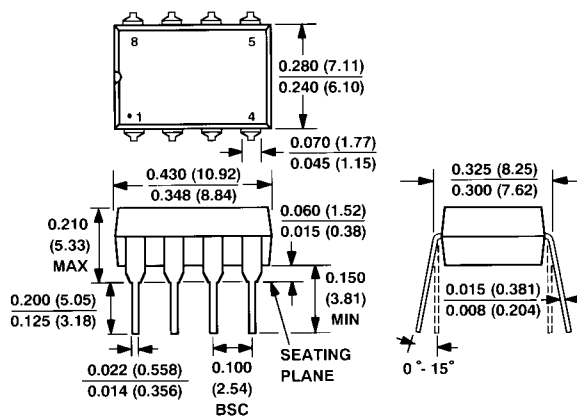
N-8
