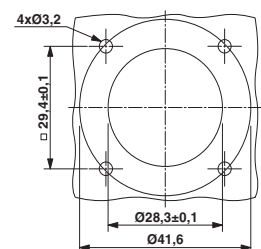
Einbaumaße
