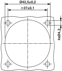
Einbaumaße
