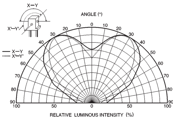
Fig. 2 Diffused type
