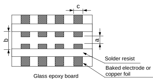
Fig.3 (in:mm)
