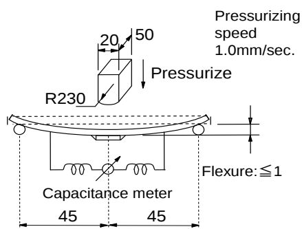
Fig.2 (in:mm)
